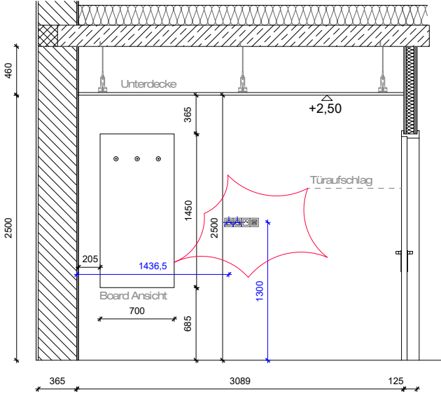
Ansicht Garderobenboard 00.04.03 - 00.06.03
