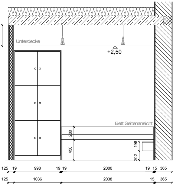
Seitenansicht Bett 00.04.02 - 00.06.02
