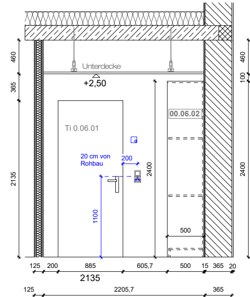
Seitenansicht Schrank 00.06.02
