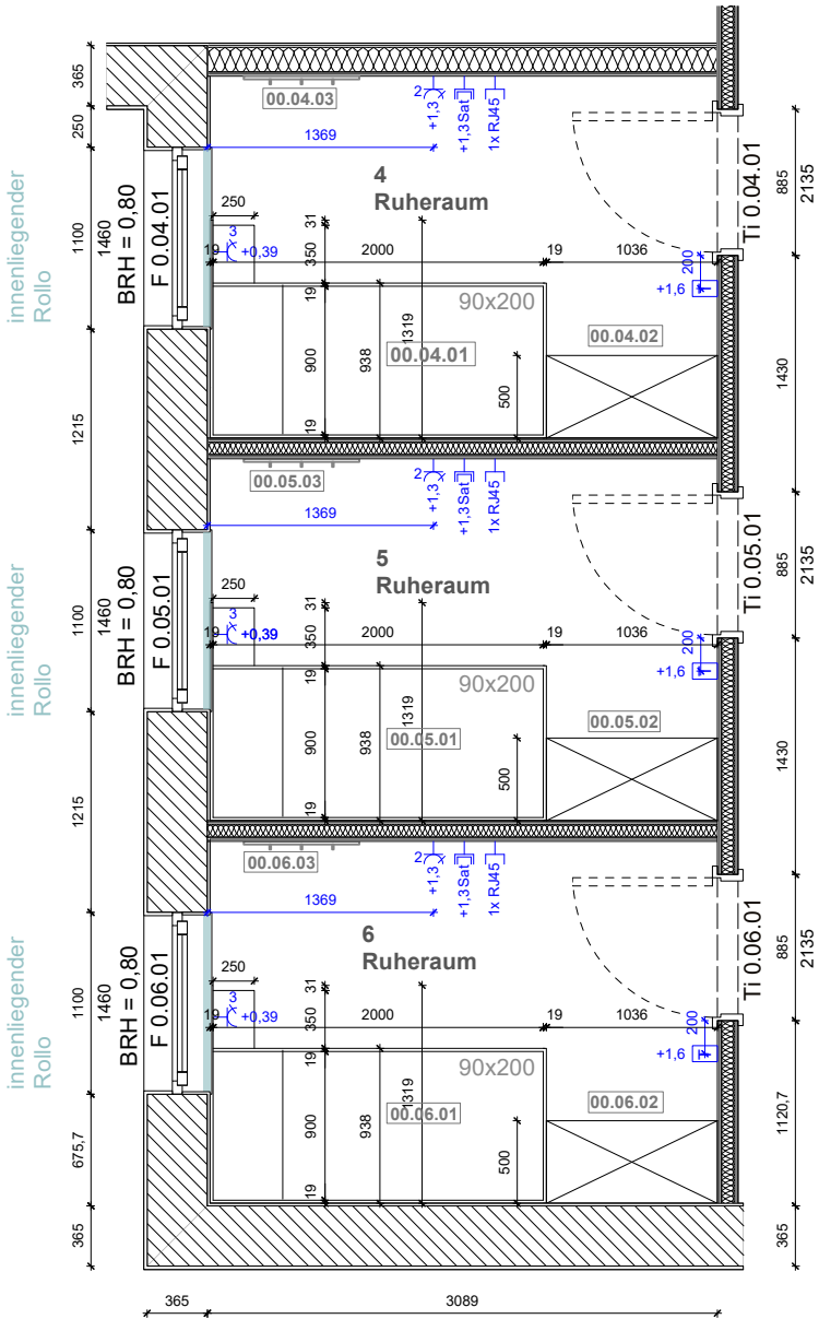
Grundriss Ruheräume Raumnr. 4-6
